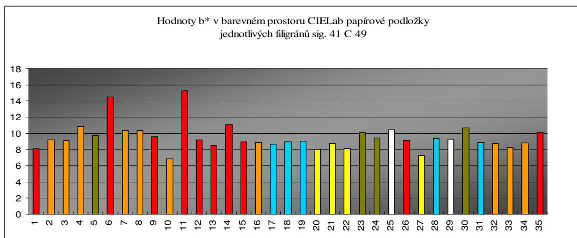
Graf. 3 Hodnoty b* papírové podložky podle jednotlivých filigránů s barevným rozlišením podle motivů (motivы uvedeny v Tab 1)
